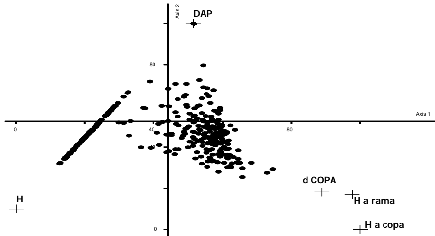
Figura No.5 Análisis DCA de la matriz general de datos. El análisis relaciona los valores de estructura en cada especie.
