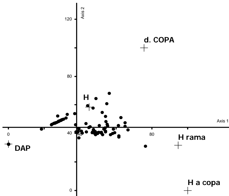
Figura No.12 Análisis DCA de la matriz general de datos. El análisis relaciona los valores estructurales de la vegetación en la totalidad de unidades de muestreo.
