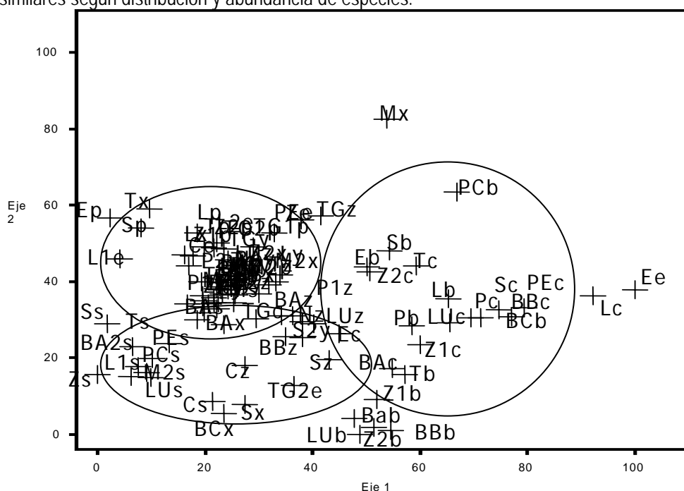
Figura No. 5 Riqueza vegetal vs. perturbación en las unidades de muestreo. Según los análisis DCA se agrupan en tres categorías: alta (a), mediana (i) y baja perturbación (b).
