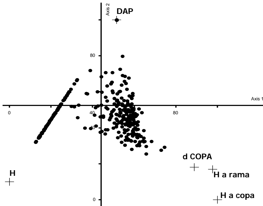
Figura No.11 Análisis DCA de la matriz general de datos. El análisis relaciona los valores de estructura en cada especie.
