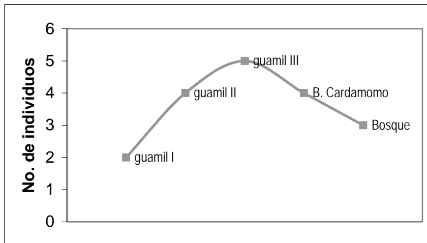
Figura No. 13 Representación idealizada de la distribución y abundancia del género Cecropia sp. en las clases vegetales. El eje “Y” indica el aumento y/o disminución de individuos en cada clase.
